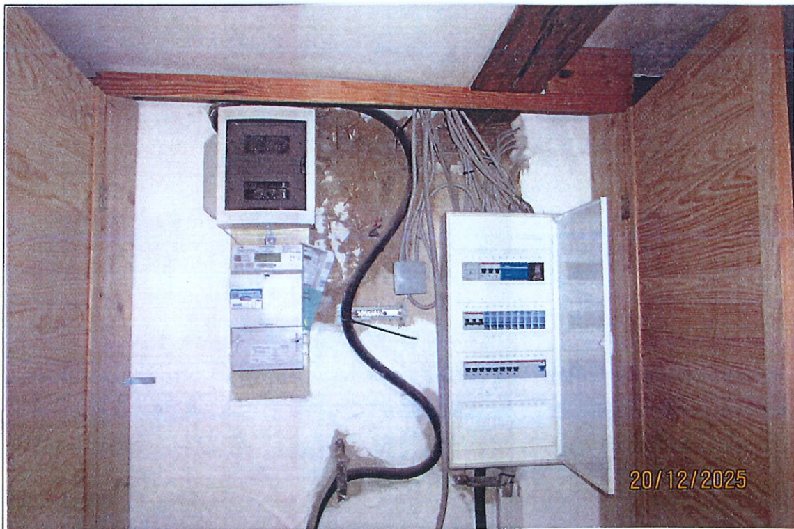
Abbildung 23: Elektrohauptanschluss mit Zähleinrichtung.
